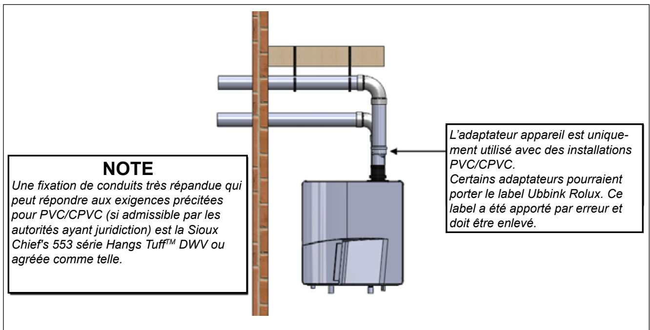
Fixation et support pour conduits PVC/CPVC recommandés
