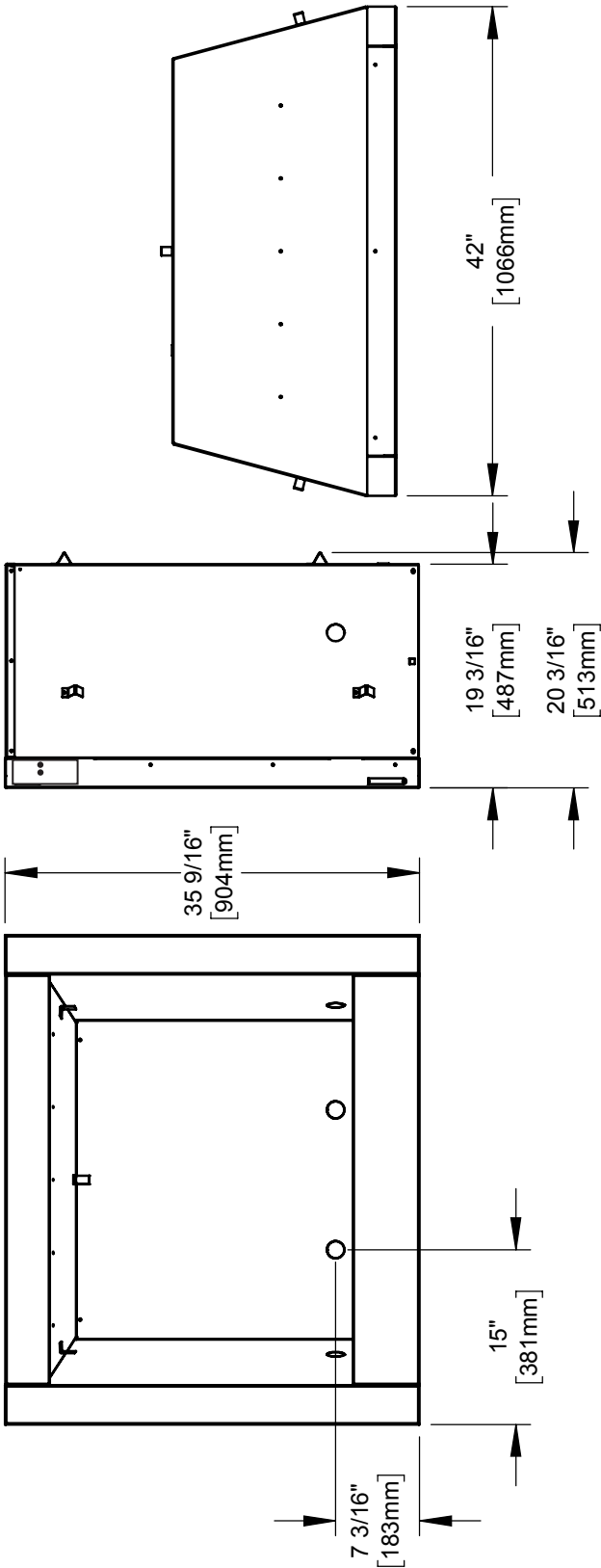
vue de face vue de côté droit vue de dessus
